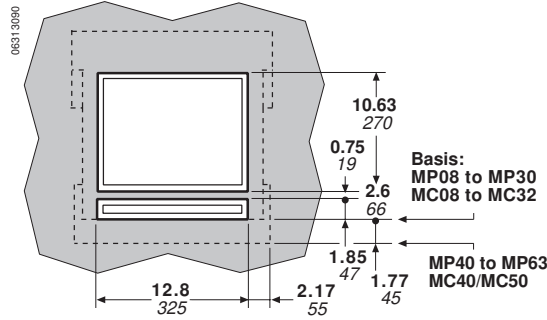
Door Cutout
